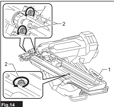
Fig.14 ► 1. Cartucho 2. Pernos
